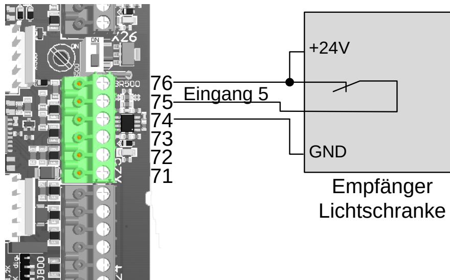
Abbildung 22: Anschluss Lichtschanke
