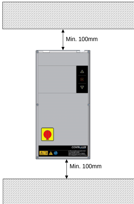
Abbildung 6: Montage großes Gehäuse
